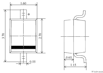
※ SOD-123（塑封长方体结构）
