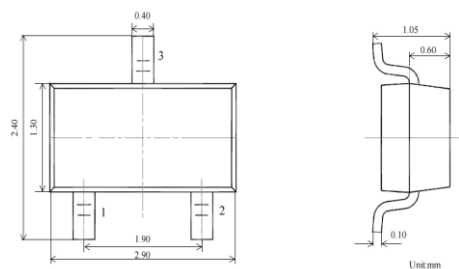
※ SOT-23（“三极管”封装形式）
