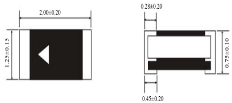
※ 厚膜片式封装(以 0805 为例)
