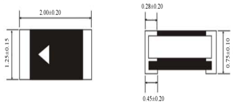
※ 厚膜片式封装(以 0805 为例)
