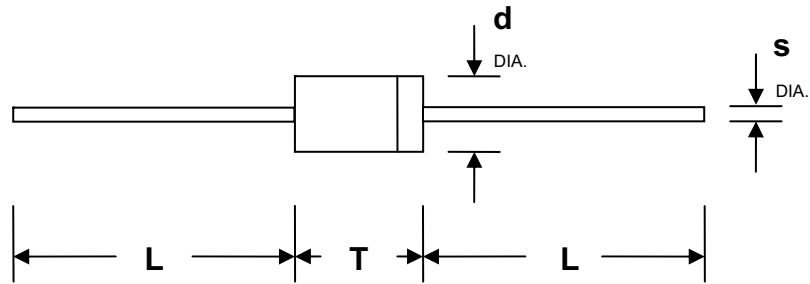
DO-204AC/DO-15
